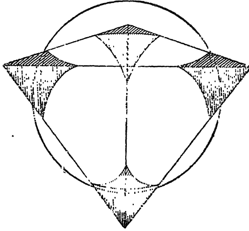
चित्र ६४—भूमंडल पर समुचित रूप से रखा हुआ चतुष्फलक
